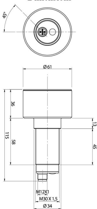
Dimensions
