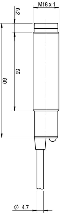
Dimensions
