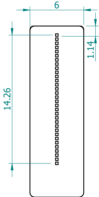
Dett. A (4:1)
