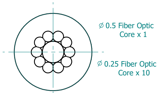
DETT. A 20:1
