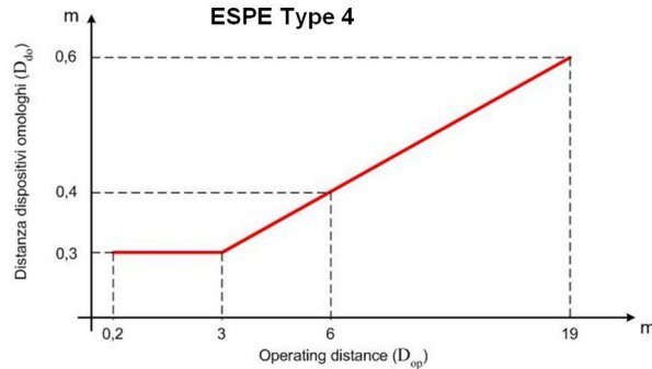
Fig 16 - ESPE Type4
