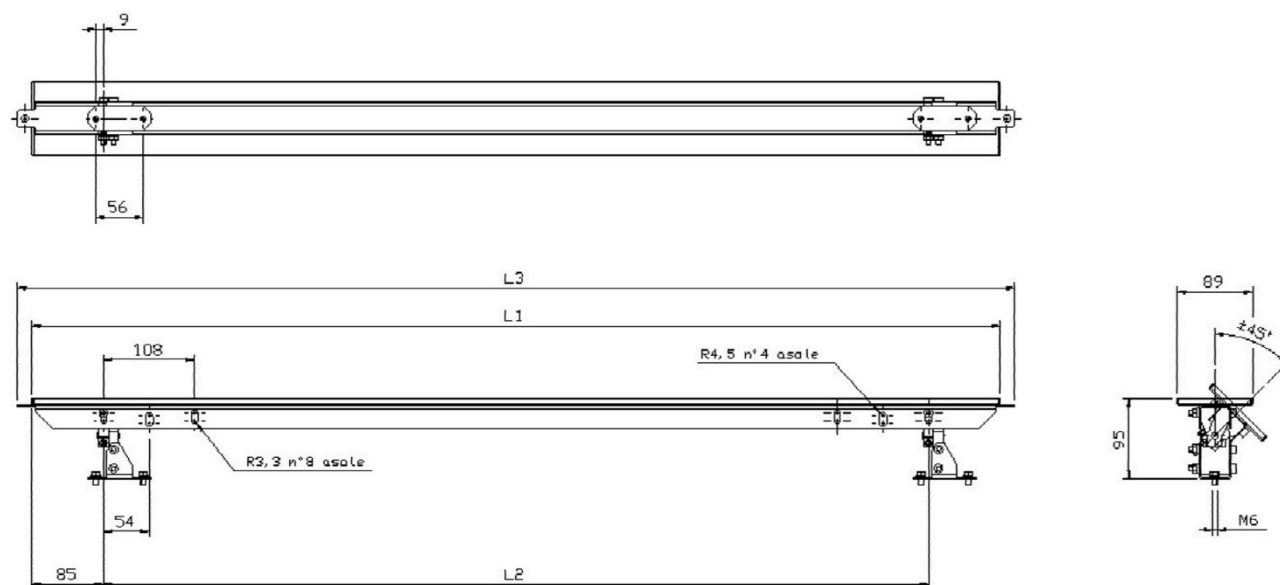
Fig 94 - Dimensions ( mm)
