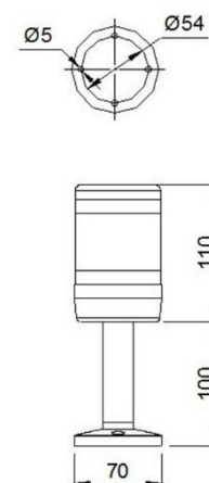
Fig 108 - Module SU-LMS-1B + LMS-1
