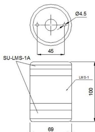
Fig 107 - Module SU-LMS-1A + LMS-1
