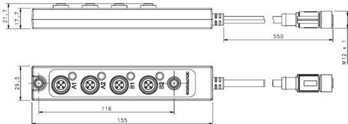
Fig 122 - Dimensions
