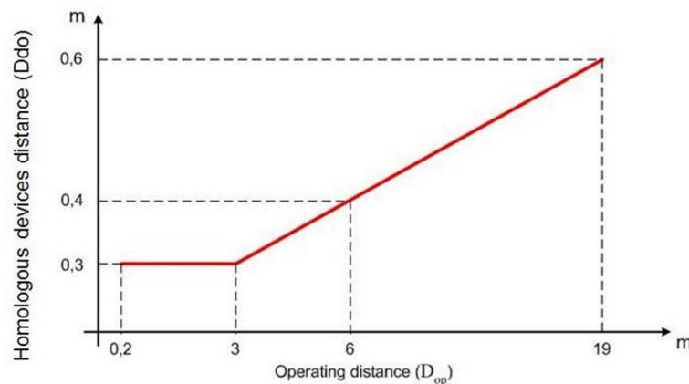
Fig 16 - ESPE Type2
