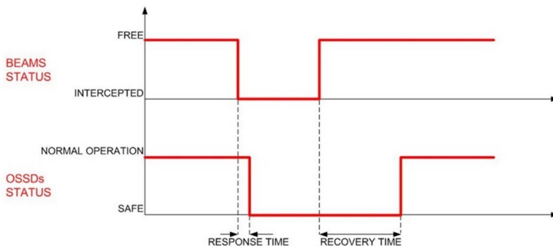
Fig 41 - Restart timings (auto)
